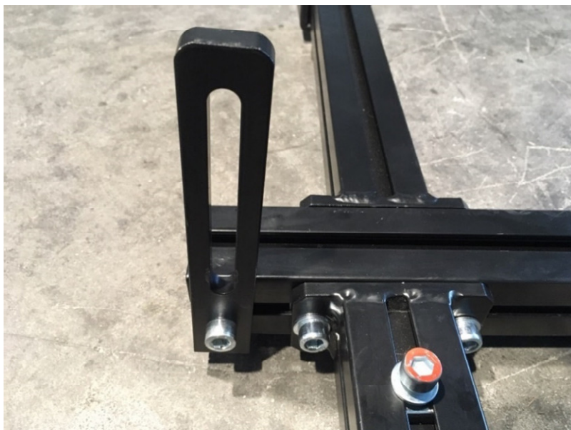
Barra Fissaggio Led, serrare tutte le viti
