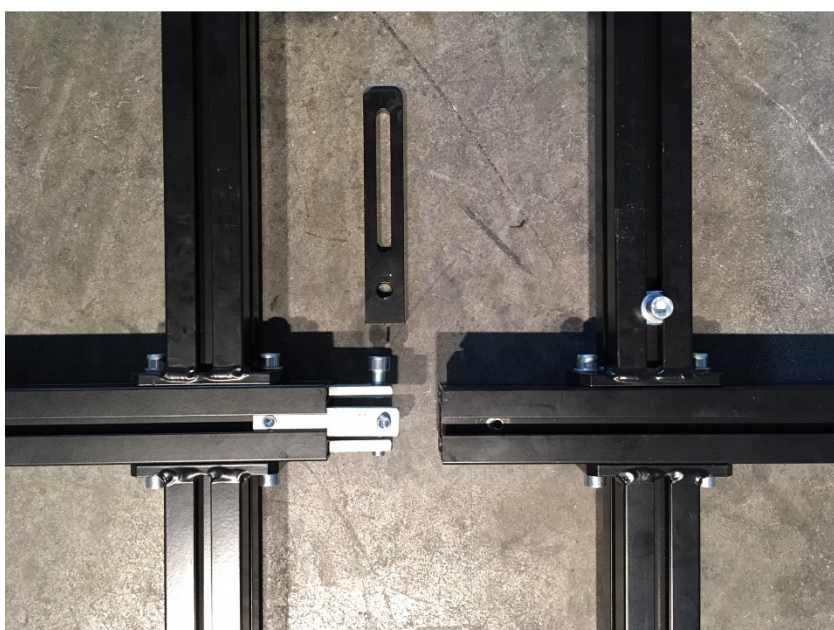
Inserire Barra Fissaggio Led (Vite Gialla)
