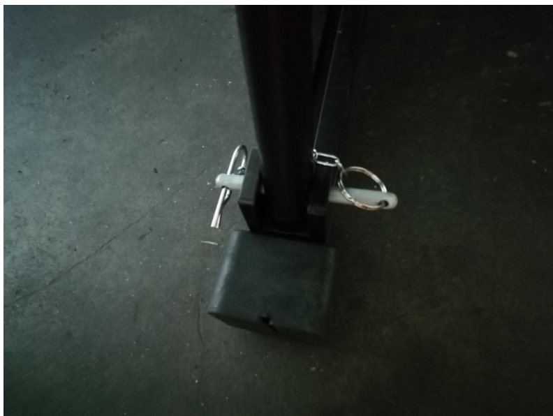
Foto dell'aggancio al piede a terra
